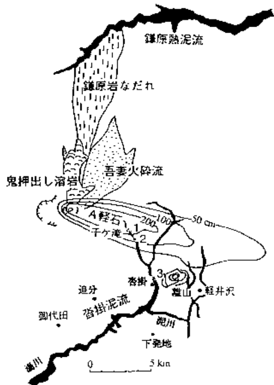
図2 浅間山麓における天明三年噴火による被害 (田村・早川, 1995)
